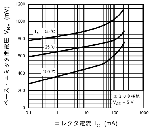
図 6.2 V_{BE} - I_C
