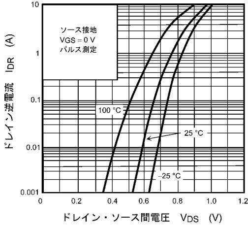
図 9.7 I_{DR} - V_{DS}
