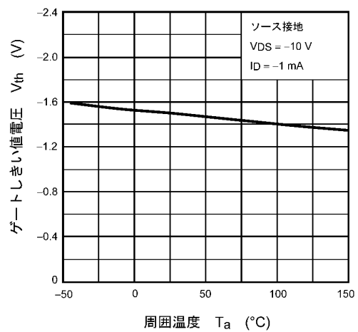
図 8.6 V_{th} - T_a
