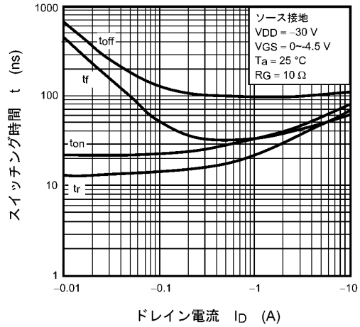
図 8.10 t - I_D
