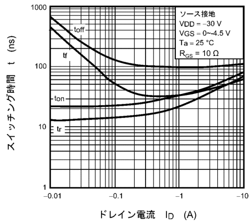
図 9.10 t - I_D
