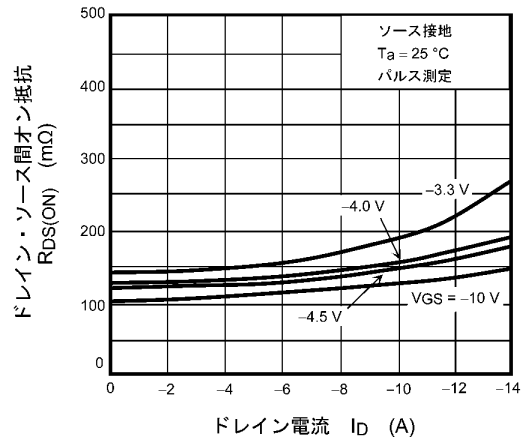
図 9.4 R_{DS(ON)} - I_D
