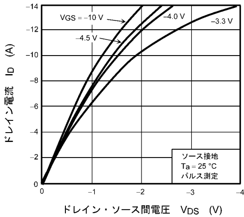
図 9.1 I_D - V_{DS}
