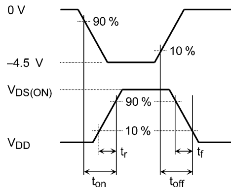
図 7.3.2 入力波形/出力波形
