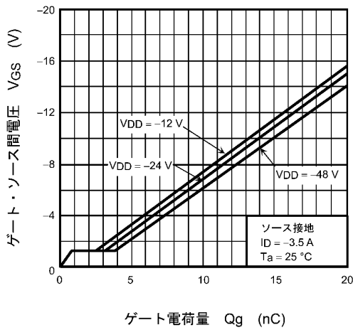
図 9.9 ダイナミック入力特性
