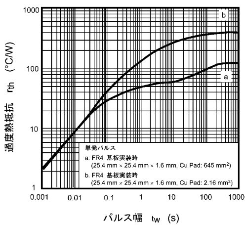
図 9.11 r_{th} - t_w
