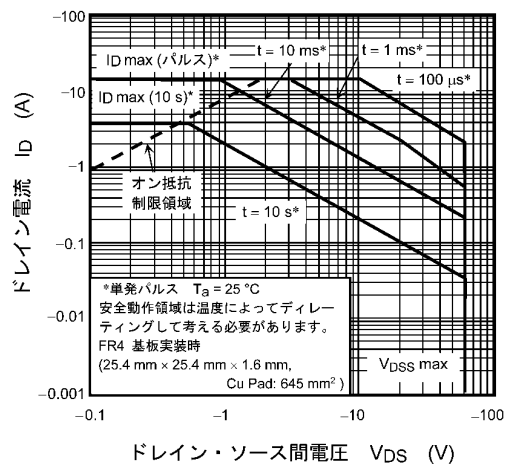
図 9.12 安全動作領域
