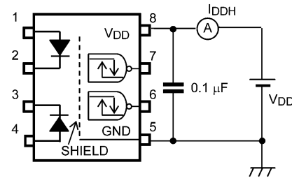
図 12.1.4 IDD H測定回路
