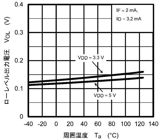
図 12.2.4 V_{OL} - T_a
