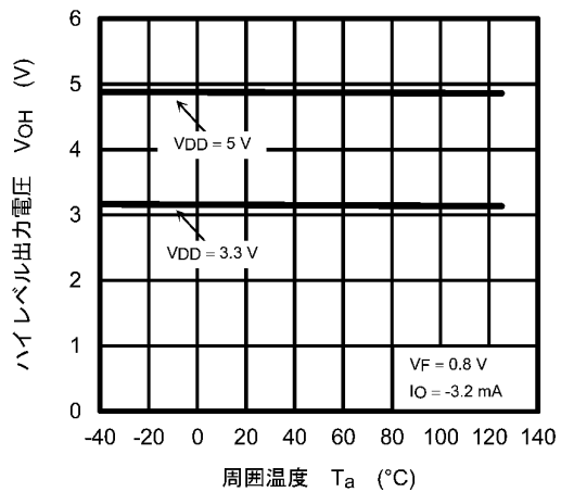
図 12.2.6 V_{OH} - T_a
