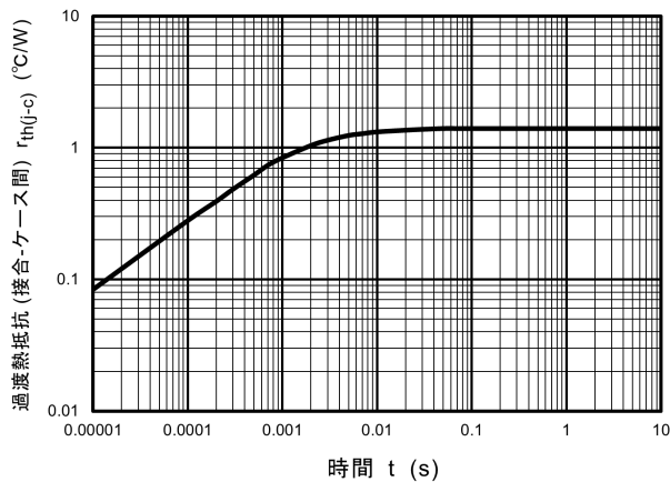
図 9.5 r_{th(j-c)} - t (最大値(保証値))
