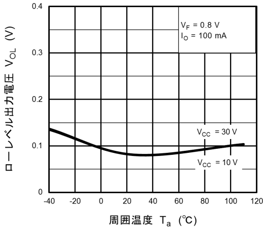
図 13.2.7 V_{OL} - T_a
