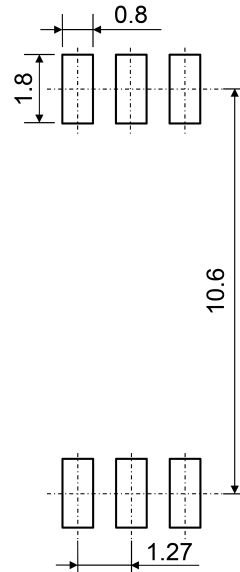
図 15.1 リードフォーミングオプション (LF4)
