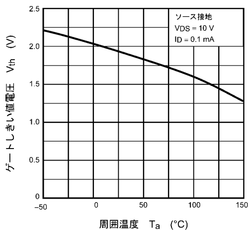
図 8.7 V_{th} - T_a
