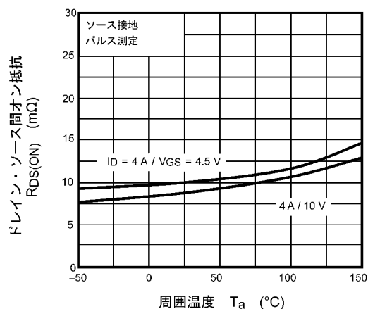
図 8.6 R_{DS(ON)} - T_a
