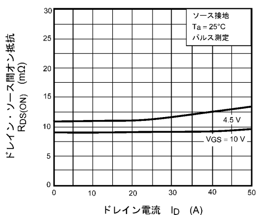
図 8.5 R_{DS(ON)} - I_D
