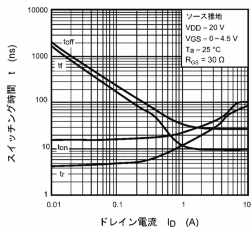
図 8.10 t - I_D
