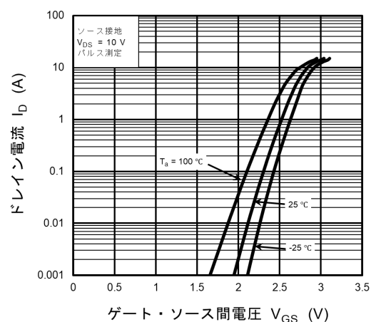
図 8.2 I_D - V_{GS}
