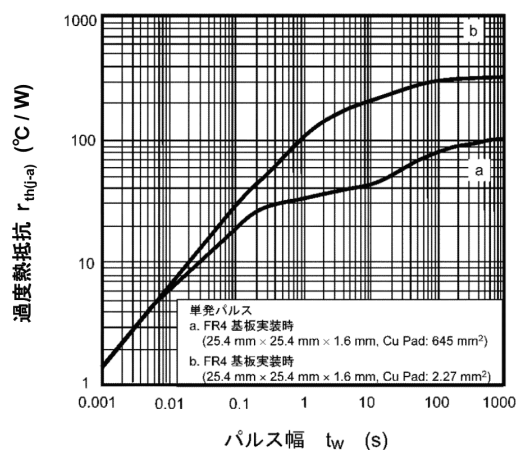
図 8.12 r_{th(j-a)} - t_w
