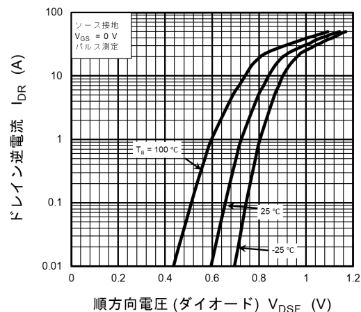
図 8.8 I_{DR} - V_{DSF}
