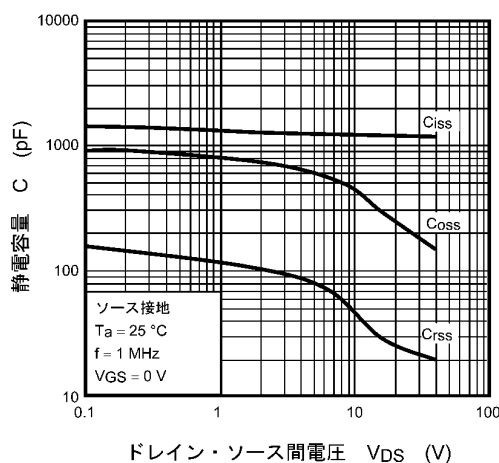
図 8.9 C - V_{DS}
