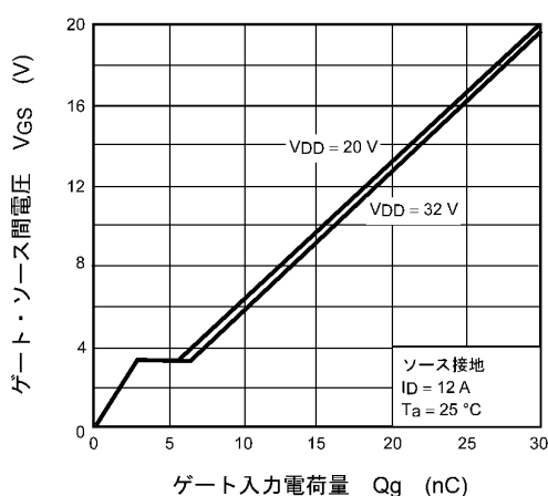
図 8.11 ダイナミック入力特性
