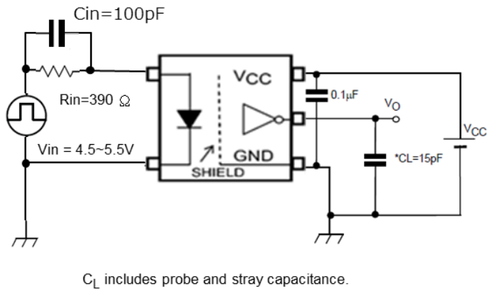
图 1 tpHL、tpLH 测定回路、波形
