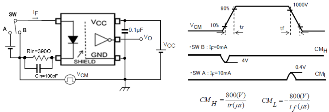
図4 コモンモード過渡耐性測定回路、波形
