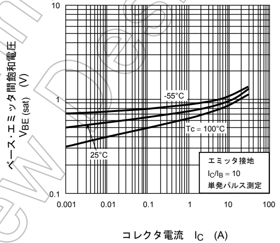
V_{BE(sat)} - I_C
