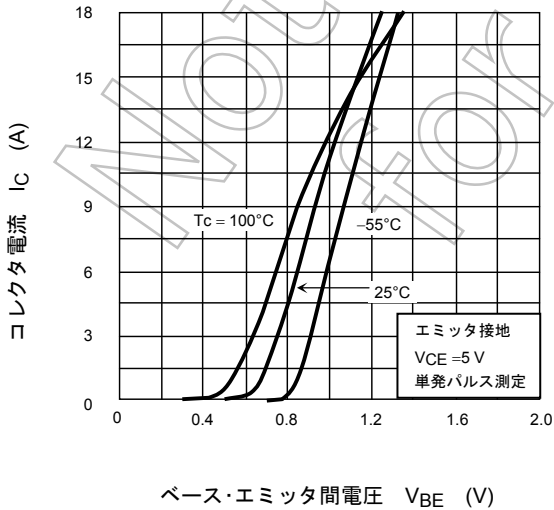
I_C - V_{BE}
