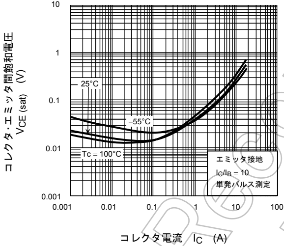
V_{CE(sat)} - I_C
