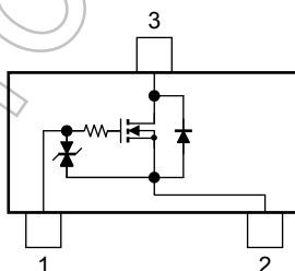
内部接続
