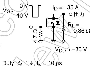
図 6.2.1 スwitchング時間の測定回路例
