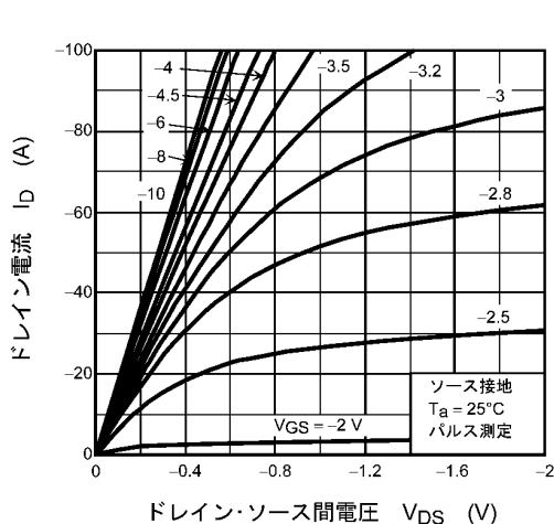
図 8.1 I_D - V_{DS}
