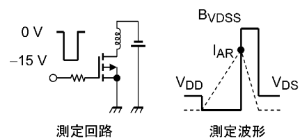
図 8.14 E_{AS} - T_{ch} (最大値 (保証値))
