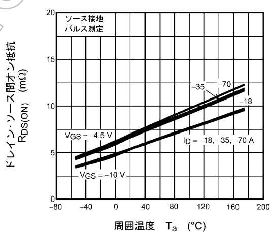
図 8.6 R_{DS(ON)} - T_a
