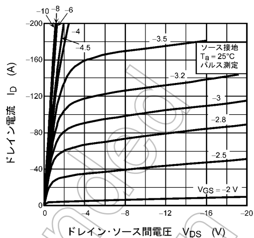
図 8.2 I_D - V_{DS}
