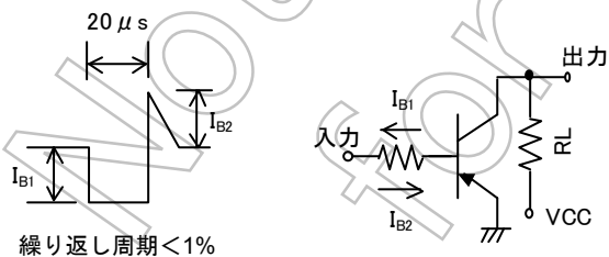
図 3. スイッチング時間測定回路
