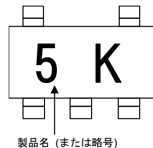
図 2. 現品表示
