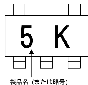
図 2. 現品表示
