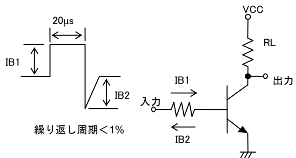
図4. スイッチング時間測定回路
