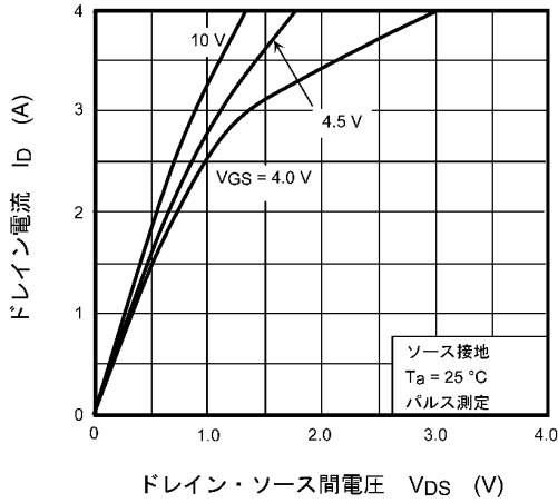
図 7.1 I_D - V_{DS}
