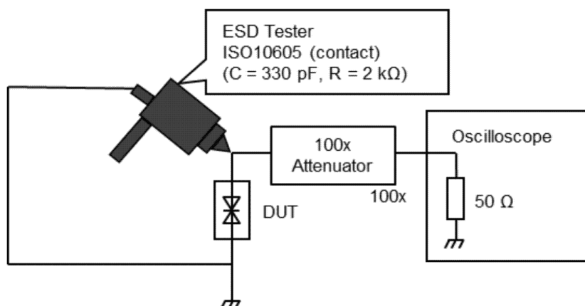
Fig. 10.5 ISO10605 (contact)
