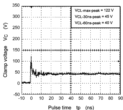
Fig. 10.1 +8 kV (ISO10605)
