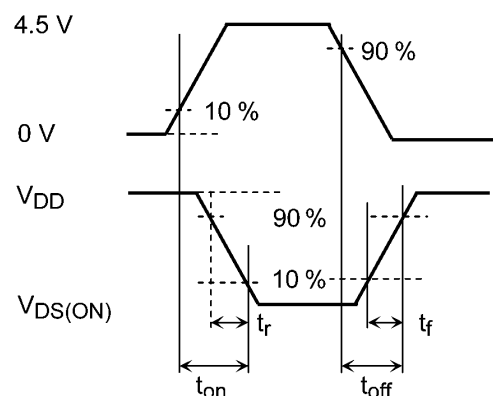
図 6.3.2 入力波形/出力波形
