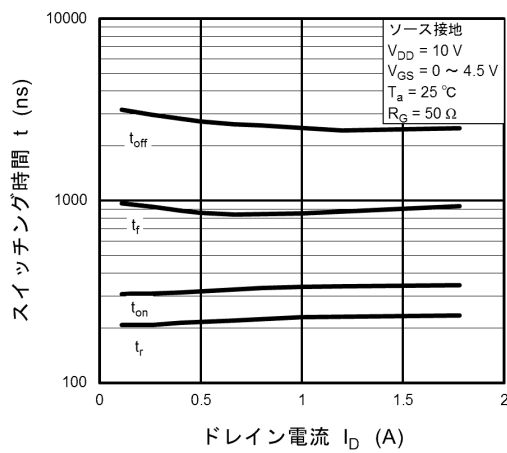
図 8.9 t - I_D
