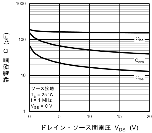
図 8.7 C - V_{DS}
