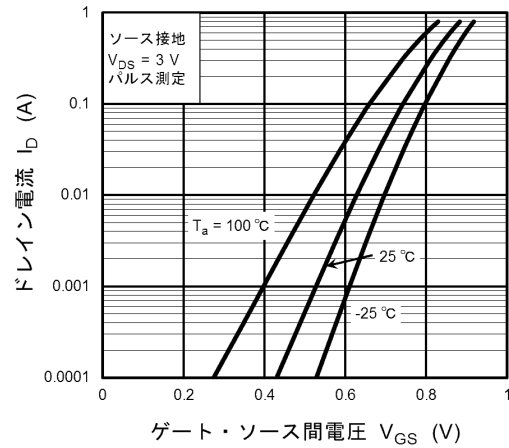
図 8.2 I_D - V_{GS}
