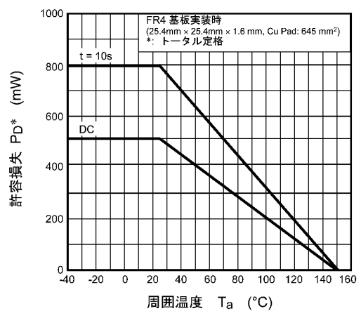
図 8.12 P_D - T_a
