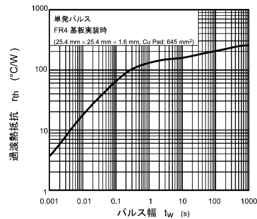
図 8.11 r_{th} - t_w
