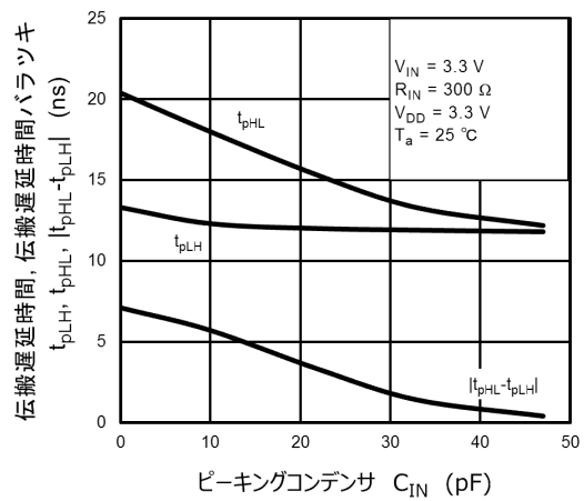
図 12.2.16 t_{pHL} , t_{pLH} , |t_{pHL} - t_{pLH}| - C_{IN}
