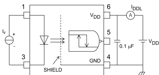
図 12.1.3 I_{DDL} 測定回路
