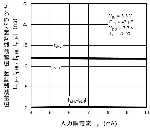
図 12.2.14 t_{pHL} , t_{pLH} , |t_{pHL} - t_{pLH}| - I_F
