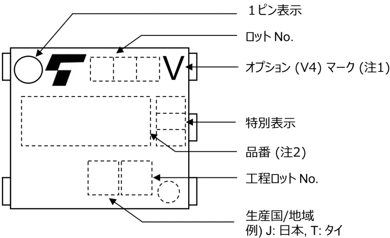
図 16.4 現品表示例
