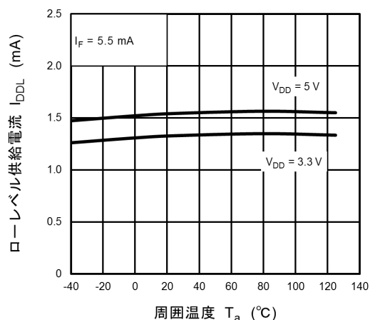
図 12.2.7 I_{DDL} - T_a
