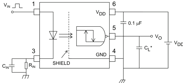
図 12.1.5 伝搬遅延時間測定回路, 波形
