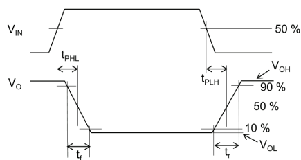
図 12.1.5 伝搬遅延時間測定回路, 波形
