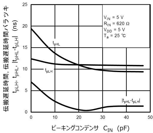
図 12.2.17 t_{pHL} , t_{pLH} , |t_{pHL} - t_{pLH}| - C_{IN}
