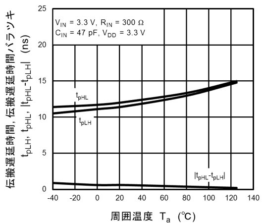
図 12.2.12 t_{pHL}, t_{pLH}, |t_{pHL} - t_{pLH}| - T_a
