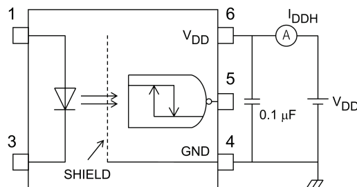
図 12.1.4 I_{DDH} 測定回路
