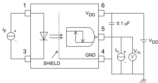
図 12.1.1 V_{OL} 測定回路
