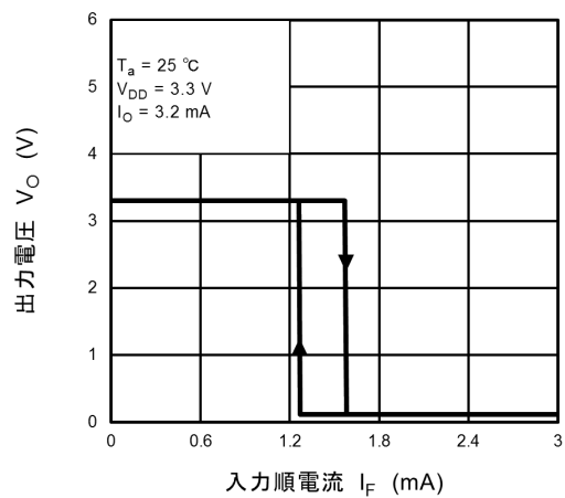
図 12.2.10 V_O - I_F
