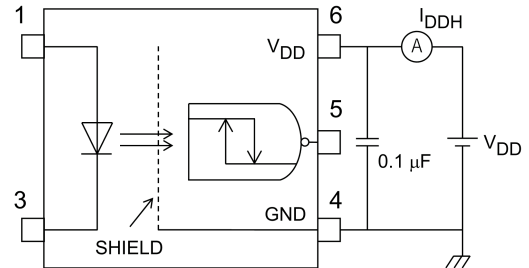
図 12.1.4 I_{DDH} 測定回路
