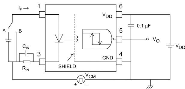
図 12.1.6 コモンモード過渡耐性測定回路, 波形
