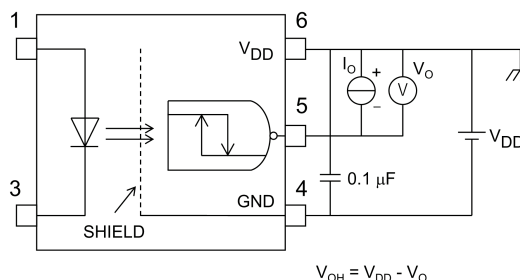
図 12.1.2 V_{OH} 測定回路
