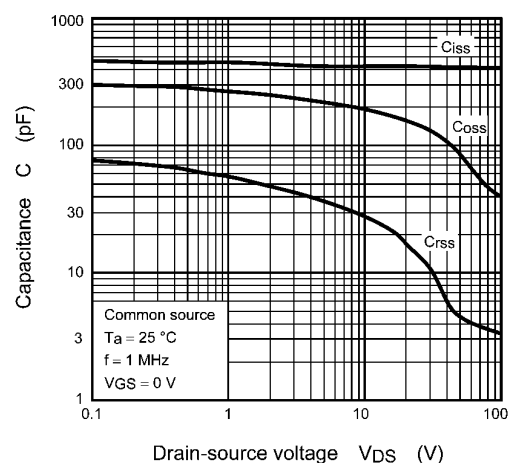
Fig. 9.8 C - V_{DS}
