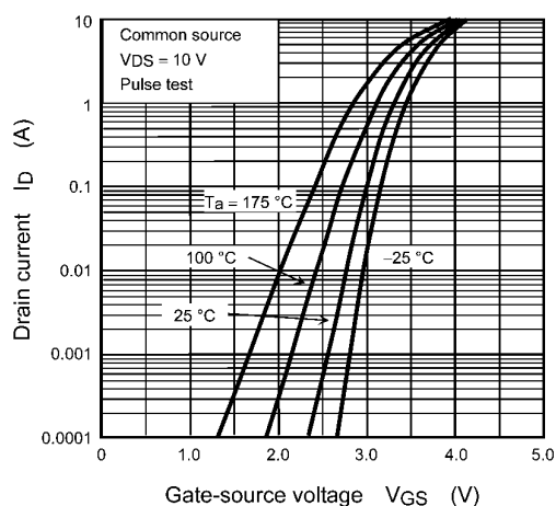
Fig. 9.2 I_D - V_{GS}
