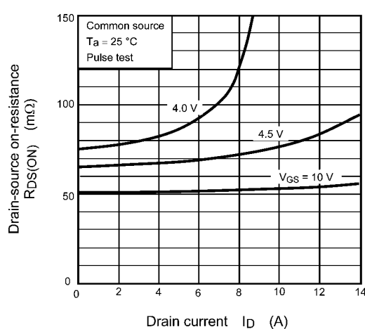
Fig. 9.4 R_{DS(ON)} - I_D
