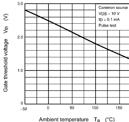
Fig. 9.6 V_{th} - T_a
