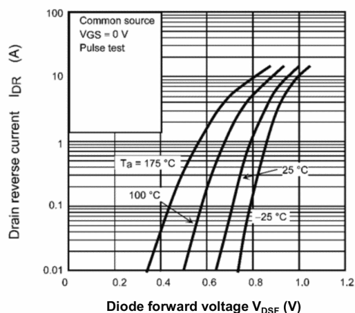
Fig. 9.7 I_{DR} - V_{DS}
