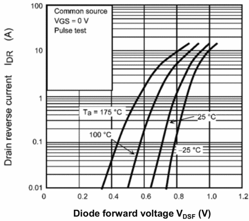
Fig. 9.7 I_{DR} - V_{DSF}
