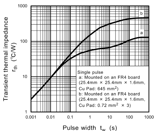
Fig. 9.12 r_{th} - t_w
