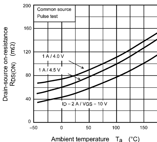
Fig. 9.5 R_{DS(ON)} - T_a
