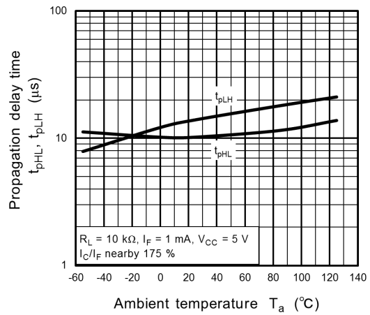
Fig. 11.16 t_{pHL}, t_{pLH} - T_a
