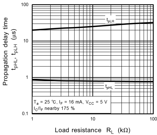
Fig. 11.15 t_{pHL}, t_{pLH} - R_L
