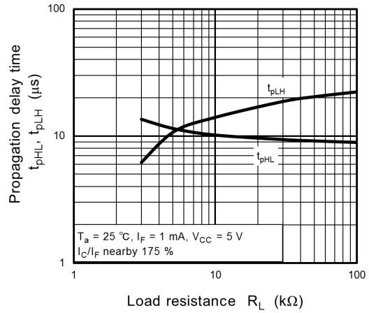
Fig. 11.14 t_{pHL}, t_{pLH} - R_L
