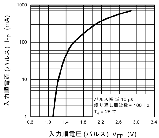
図 11.6 I_{FP} - V_{FP}
