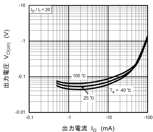
図 7.5 V_{O(on)} - I_O
