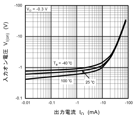
図 7.1 V_{I(on)} - I_O
