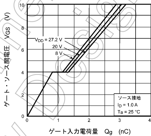
図 7.10 ダイナミック入力特性
