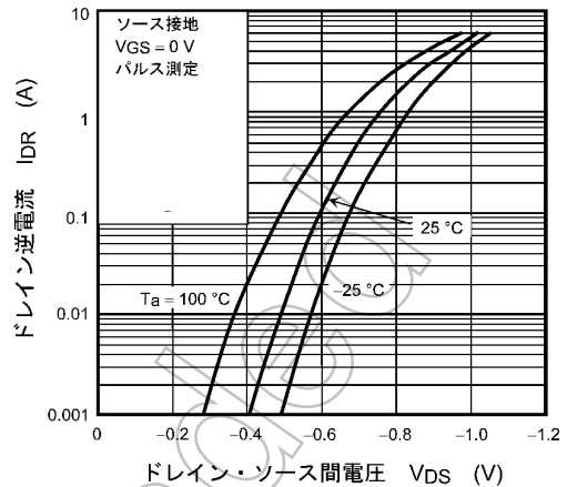
図 7.8 I_{DR} - V_{DS}
