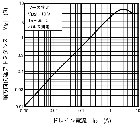
図 7.7 |Y_{fs}| - I_D
