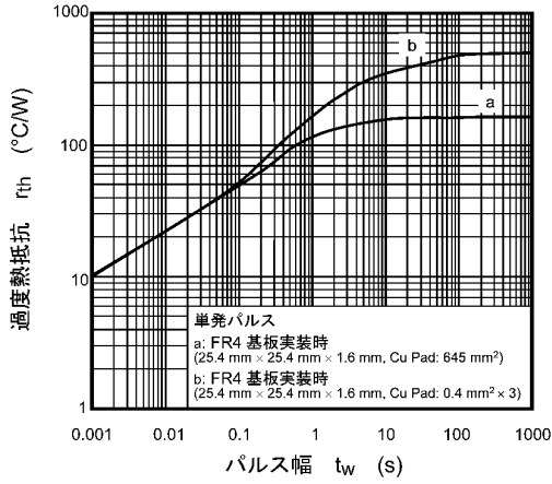
図 7.13 r_{th} - t_w (Zener)
