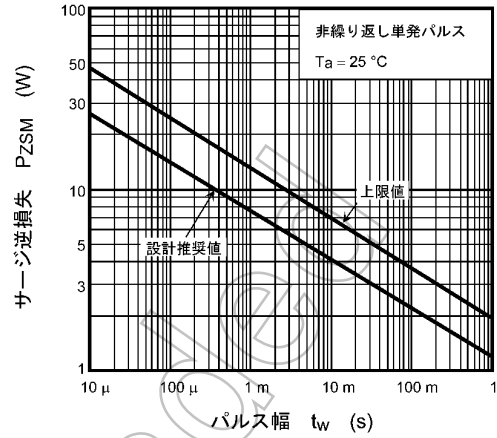
図 7.14 P_{zsm} - t
