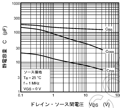
図 7.9 C - V_{DS}
