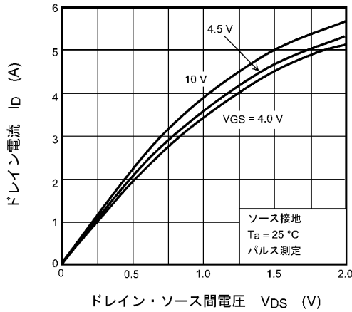
図 7.1 I_D - V_{DS}
