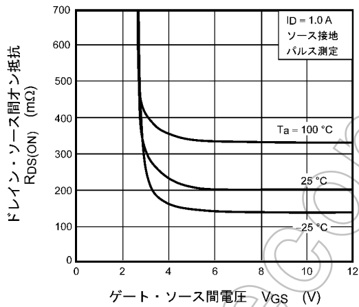
図 7.3 R_{DS(ON)} - V_{GS}
