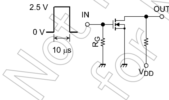
図 5.3.1 スwitchング時間の測定回路
