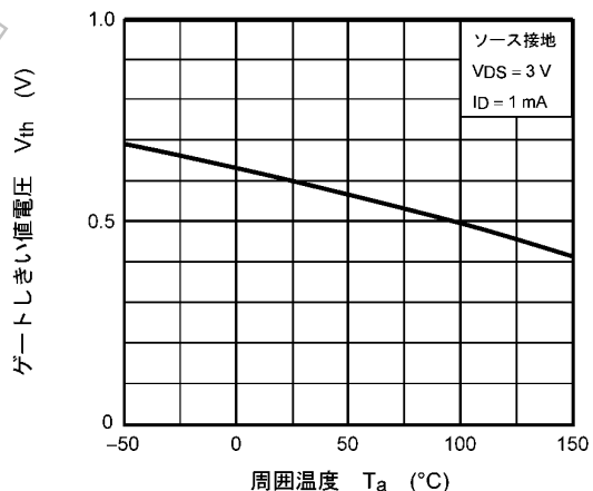
図 8.6 V_{th} - T_a
