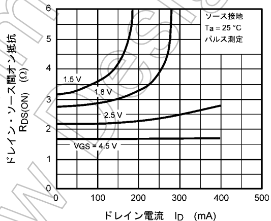
図 8.4 R_{DS(ON)} - I_D
