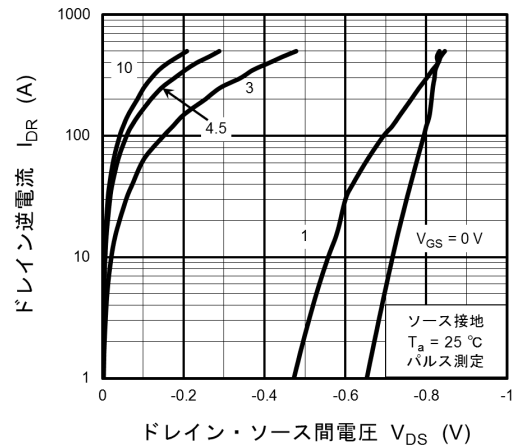
図 8.6 I_{DR} - V_{DS}
