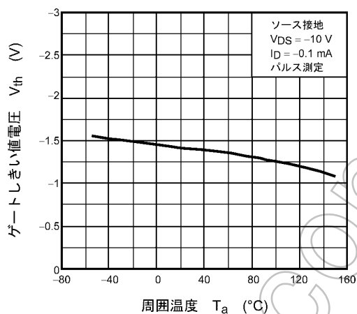
図 8.1.9 V_{th} - T_a
