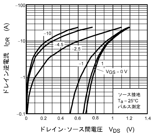
図 8.1.7 I_{DR} - V_{DS}
