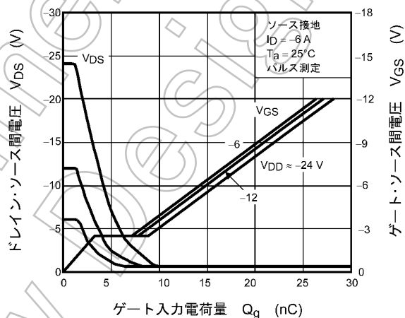
図 8.1.10 ダイナミック入出力特性
