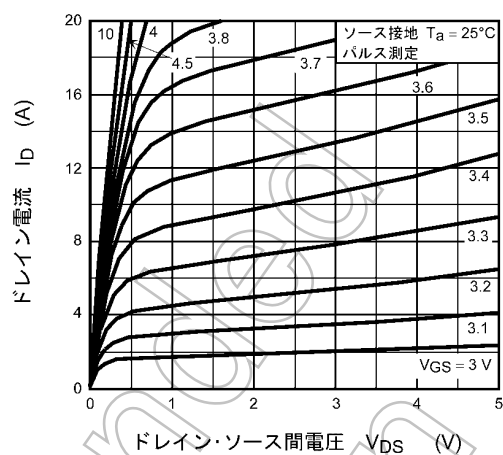
図 8.2.2 I_D - V_{DS}
