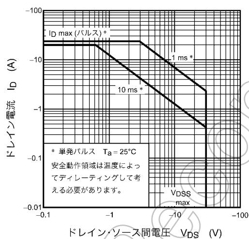
図 8.1.13 安全動作領域 (最大値 (保証値))
