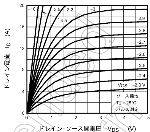
図 8.1.2 I_D - V_{DS}
