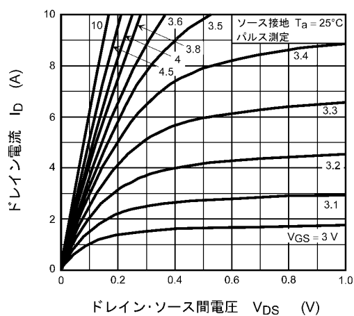
図 8.2.1 I_D - V_{DS}
