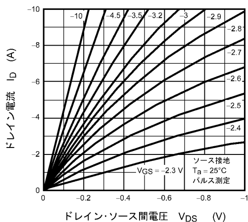
図 8.1.1 I_D - V_{DS}
