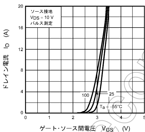
図 8.2.3 I_D - V_{GS}
