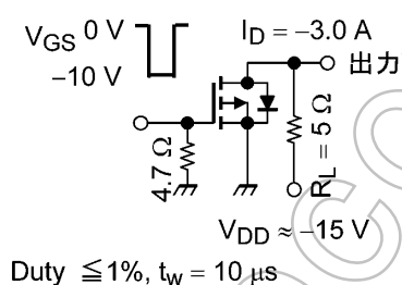
図 6.2.1 スwitchング時間の測定回路例 (P-ch) 図 6.2.2 スwitchング時間の測定回路例 (N-ch)
