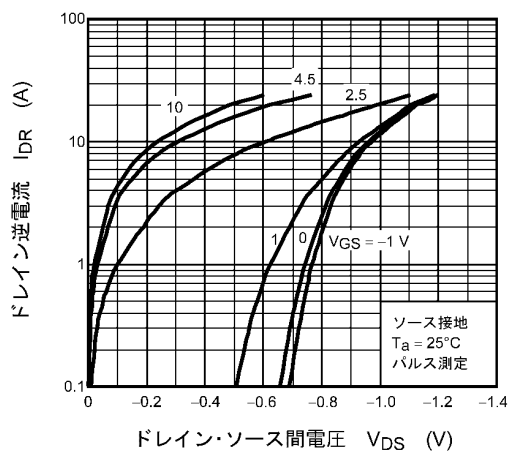
図 8.2.7 I_{DR} - V_{DS}
