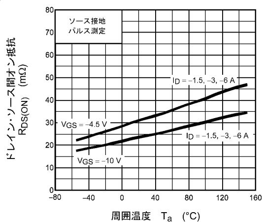
図 8.1.6 R_{DS(ON)} - T_a
