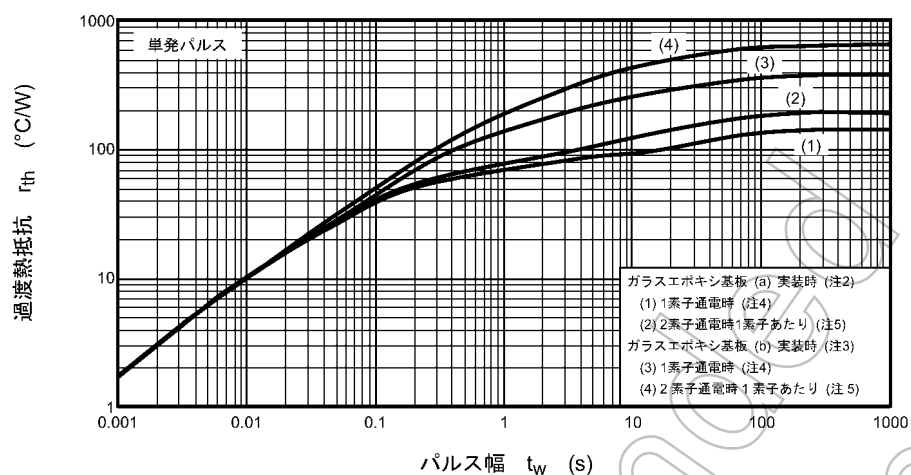
図 8.2.12 r_{th} - t_w (最大値 (保証値))
