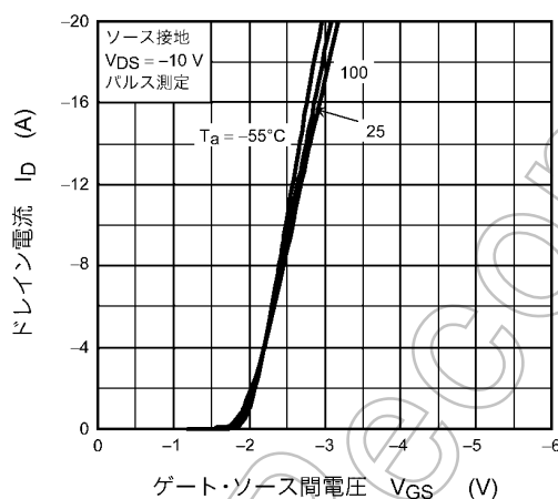
図 8.1.3 I_D - V_{GS}
