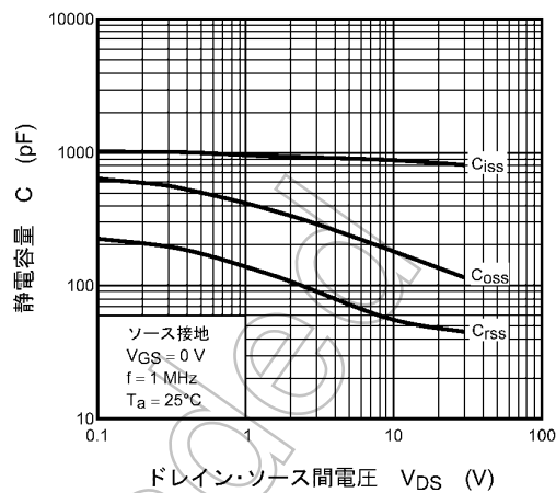
図 8.2.8 静電容量 - V_{DS}
