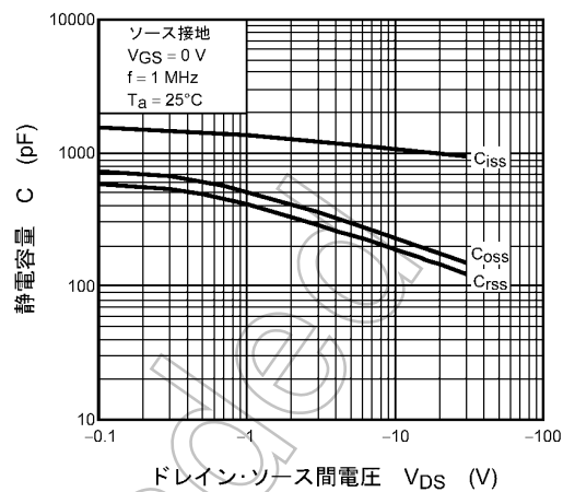
図 8.1.8 静電容量 - V_{DS}
