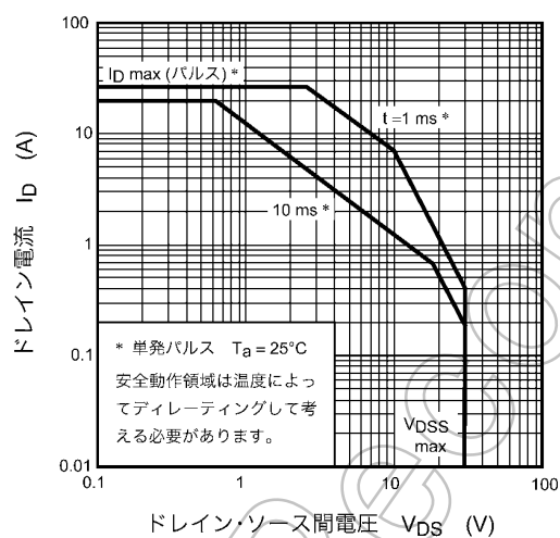
図 8.2.13 安全動作領域 (最大値 (保証値))
