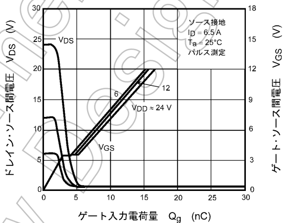
図 8.2.10 ダイナミック入出力特性
