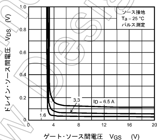
図 8.2.4 V_{DS} - V_{GS}
