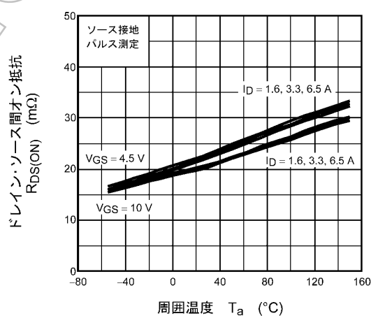
図 8.2.6 R_{DS(ON)} - T_a
