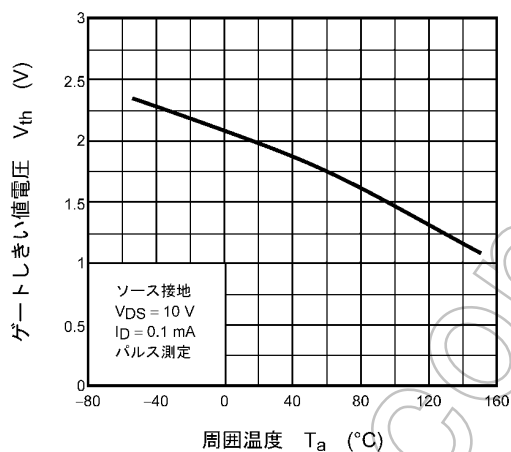
図 8.2.9 V_{th} - T_a
