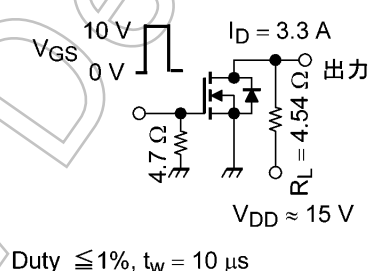
図 6.2.1 スwitchング時間の測定回路例 (P-ch) 図 6.2.2 スwitchング時間の測定回路例 (N-ch)
