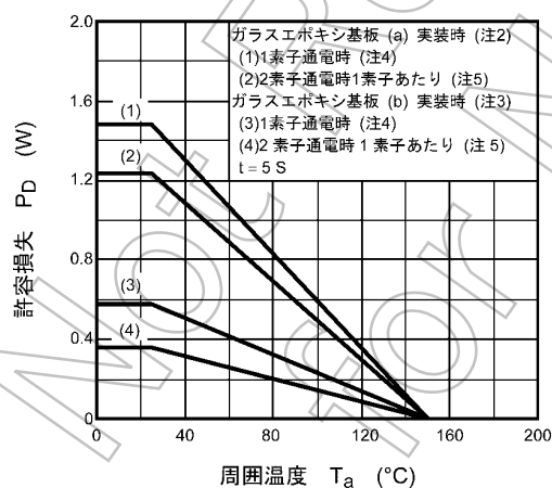
図 8.1.11 P_D - T_a (最大値 (保証値))
