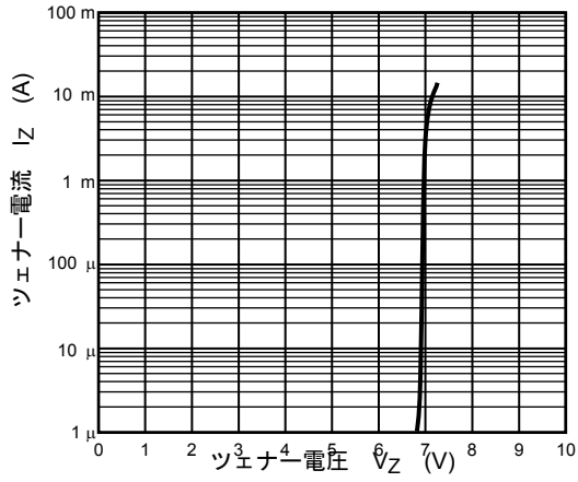
I_Z - V_Z
