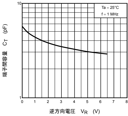
C_T - V_R
