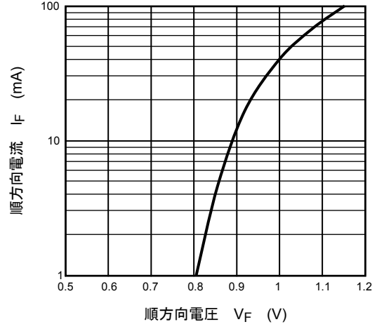
I_F - V_F
