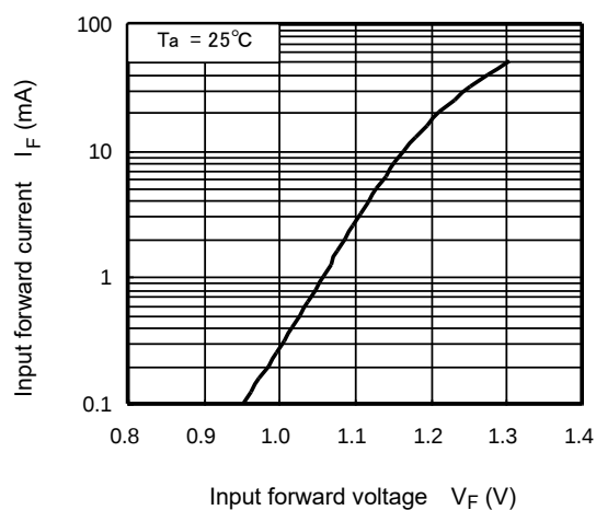
Fig.12.3 I_F - V_F
