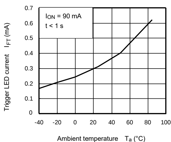
Fig.12.6 I_{FT} - T_a
