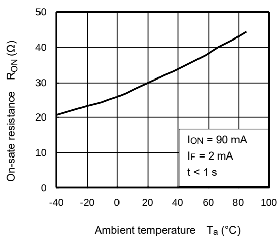
Fig.12.5 R_{ON} - T_a
