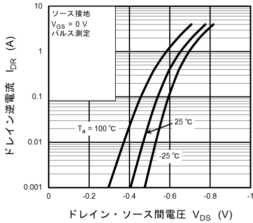
図 9.7 I DR - V DS
