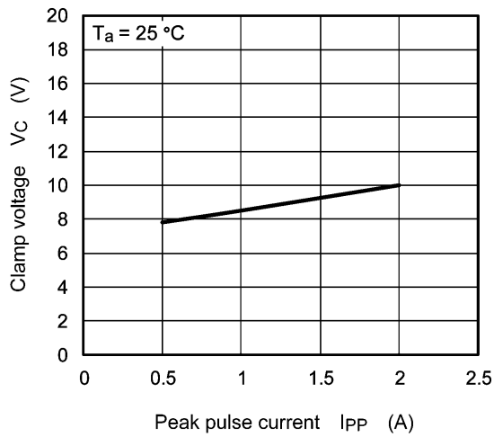
図 6.3.1 V_C - I_{PP}
