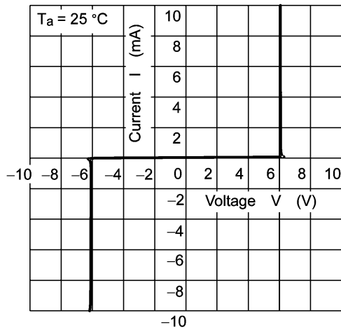
図 9.1 I - V
