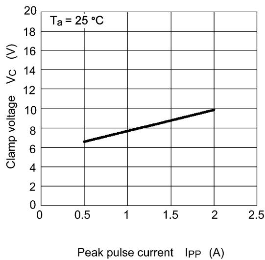
図 6.3.1 V_C - I_{PP}
