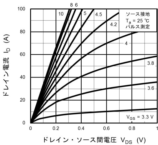
図 8.1 I_D - V_{DS}
