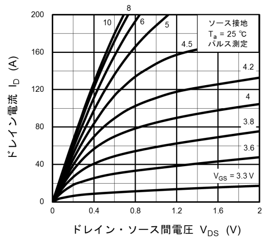
図 8.2 I_D - V_{DS}
