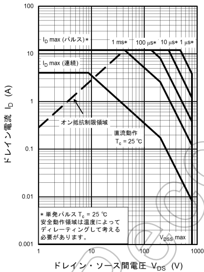
図 8.14 安全動作領域 (最大値 (保証値))
