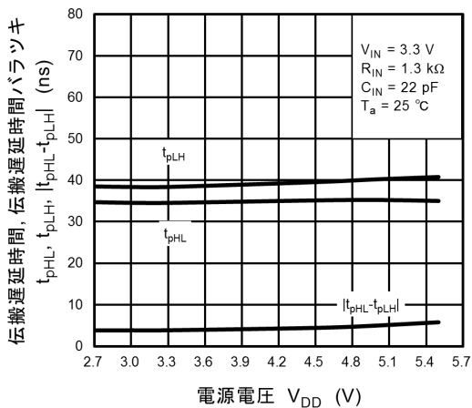
図 12.2.16 t_{pHL} , t_{pLH} , |t_{pHL} - t_{pLH}| - V_{DD}
