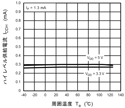
図 12.2.8 I_{DDH} - T_a
