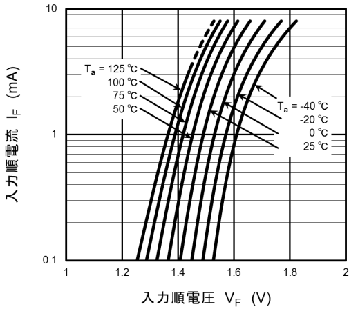
図 12.2.1 I_F - V_F
