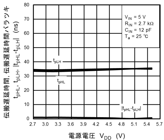
図 12.2.17 t_{pHL} , t_{pLH} , |t_{pHL} - t_{pLH}| - V_{DD}
