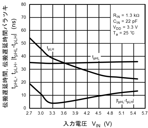
図 12.2.14 t_{pHL} , t_{pLH} , |t_{pHL} - t_{pLH}| - V_{IN}
