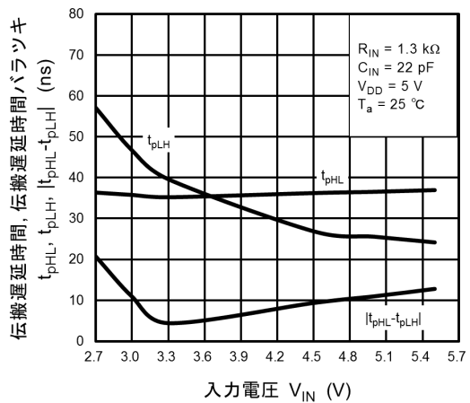
図 12.2.15 t_{pHL} , t_{pLH} , |t_{pHL} - t_{pLH}| - V_{IN}
