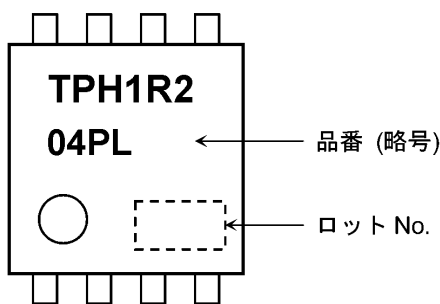
図 7.1 現品表示
