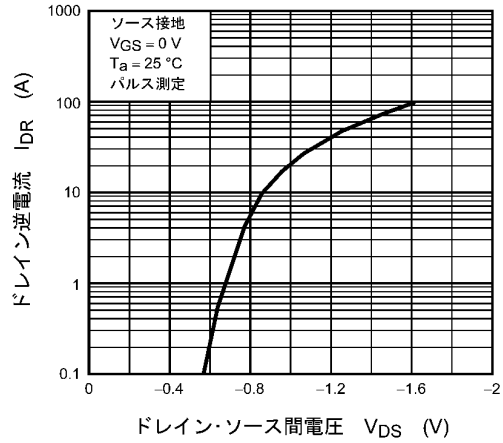
図 8.8 I DR - V DS
