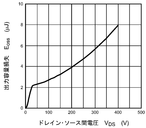
図 8.10 E oss - V DS
