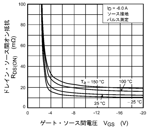
図 8.4 R_{DS(ON)} - V_{GS}
