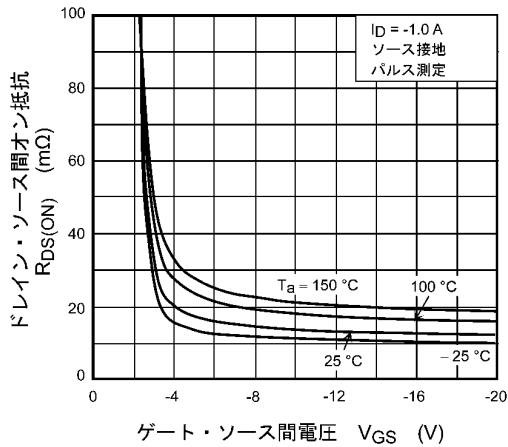
図 9.3 R_{DS(ON)} - V_{GS}
