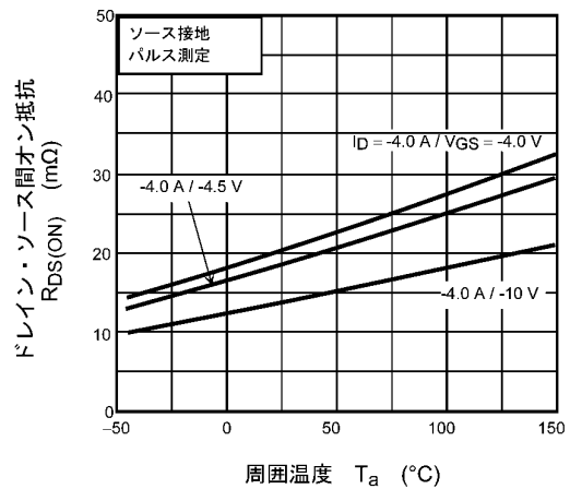
図 9.6 R_{DS(ON)} - T_a
