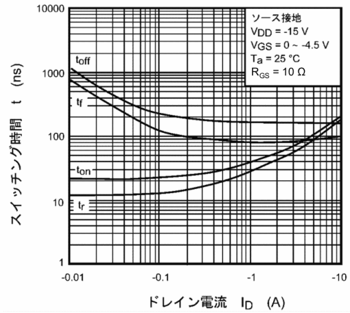
図 9.10 t - I_D
