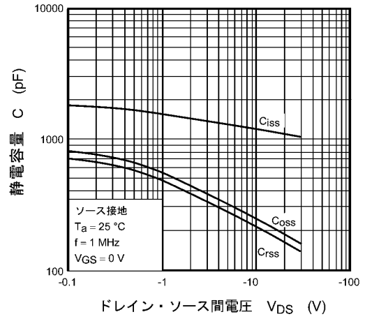
図 9.8 C - V_{DS}
