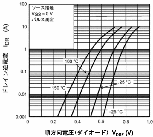
図 9.11 I_{DR} - V_{DSF}
