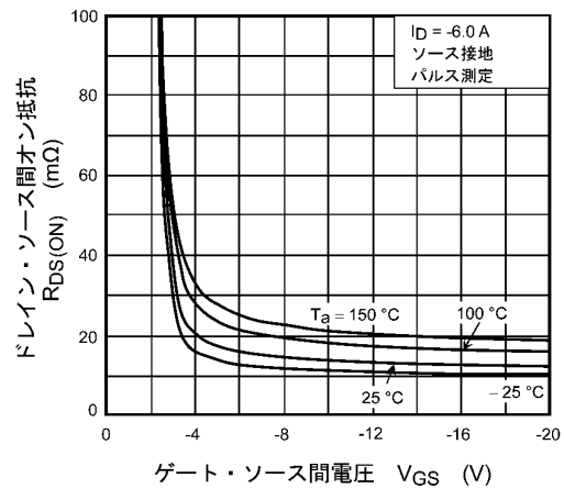
図 9.4 R_{DS(ON)} - V_{GS}
