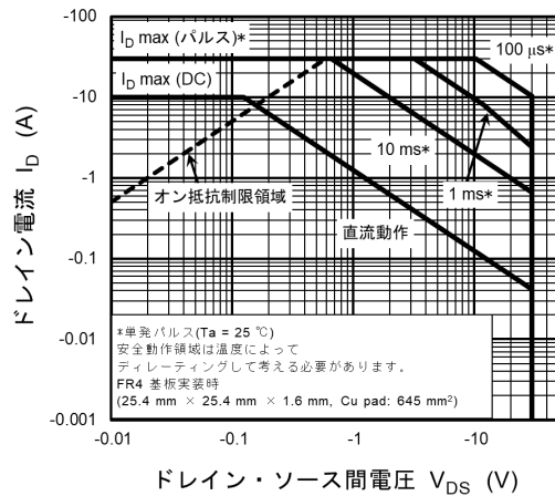
図 9.12 安全動作領域
