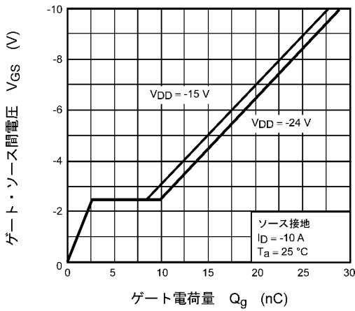
図 9.9 ダイナミック入力特性
