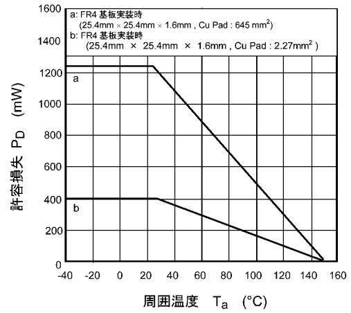
図 9.14 P_D - T_a
