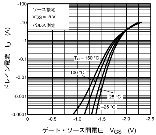
図 9.2 I_D - V_{GS}
