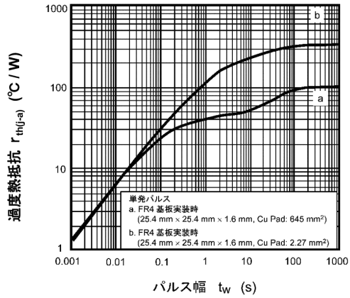
図 9.13 r_{th(j-a)} - t_w
