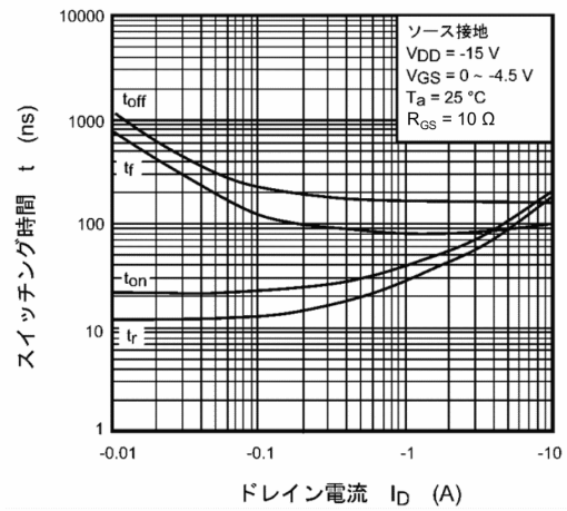
図 8.10 t - I_D
