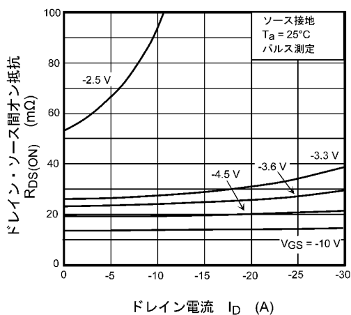
図 9.5 R_{DS(ON)} - I_D
