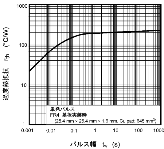
図 8.11 r th - t w
