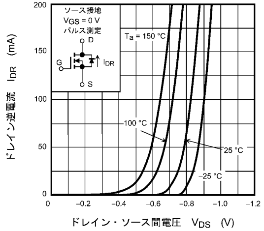
図 8.8 I DR - V DS
