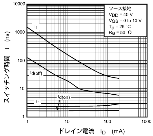
図 8.10 t - I D
