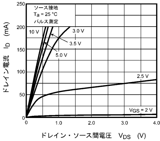
図 8.1 I_D - V_{DS}
