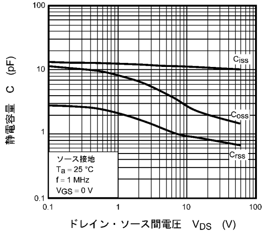
図 8.7 C - V DS
