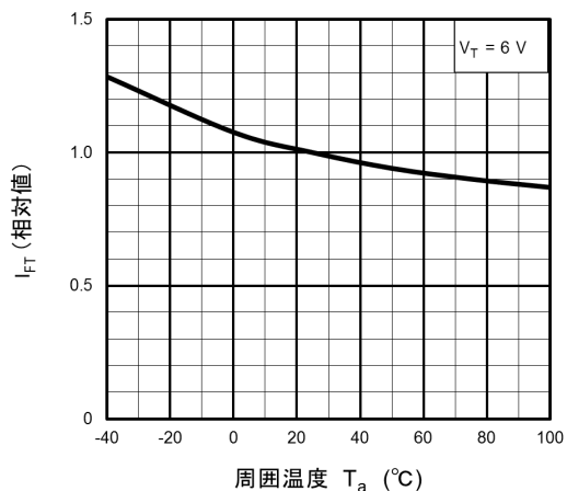
図 12.7 相対 I_{FT} - T_a
