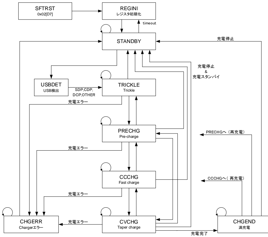
Figure: 22 Charger ファンクションフローチャート
