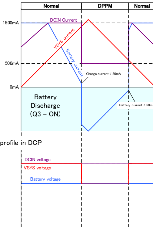
Figure: 14 DCP, Other 検出時のタイミングチャート (DCIN 電流制限 = 1500 mA 設定)
