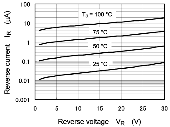
図 9.2 I_R - V_R
