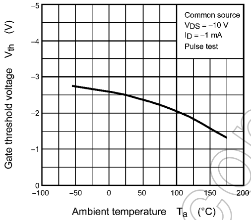
Fig. 9.9 V_{th} - T_a
