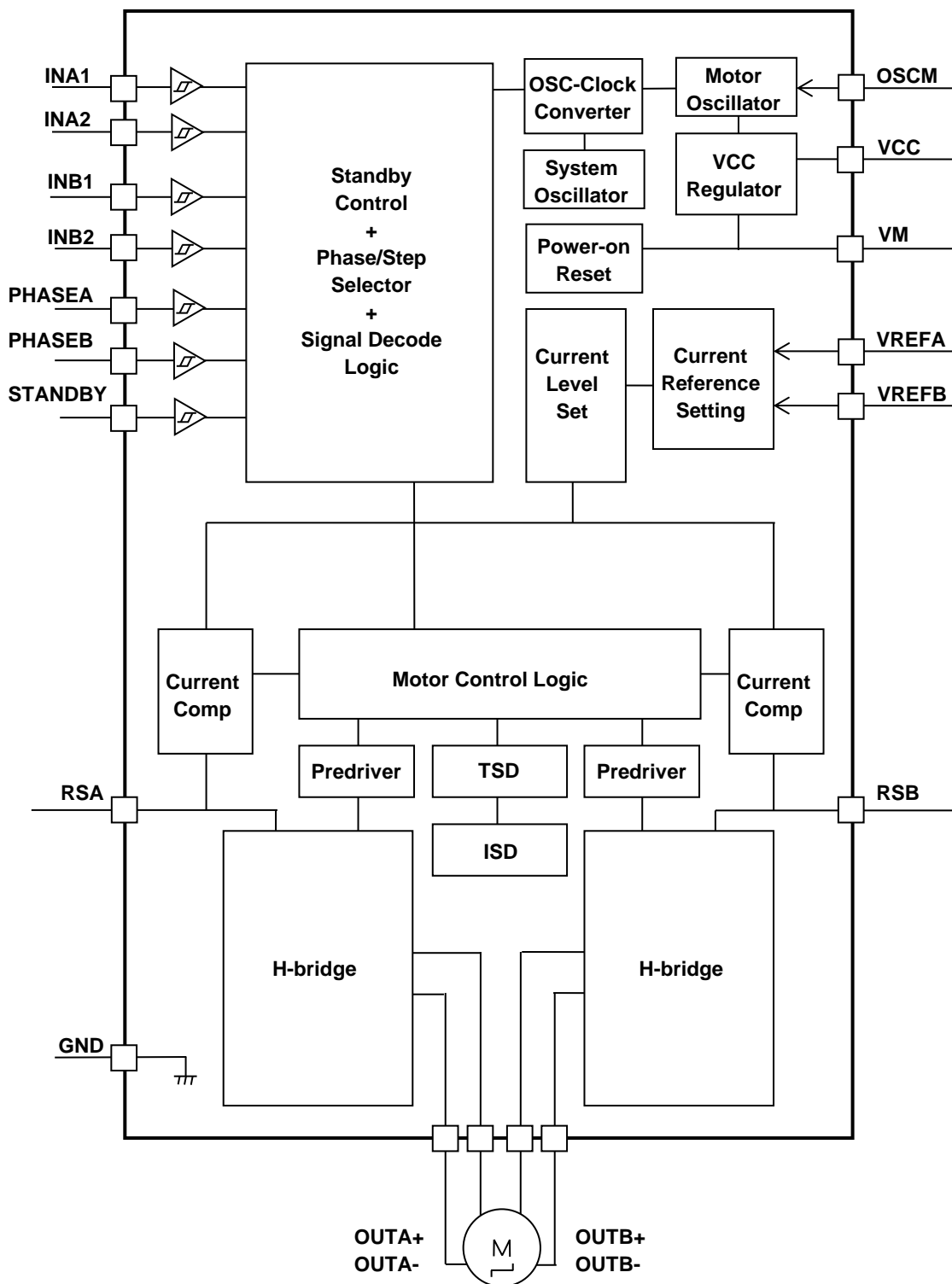
図 3.1 ブロック図
