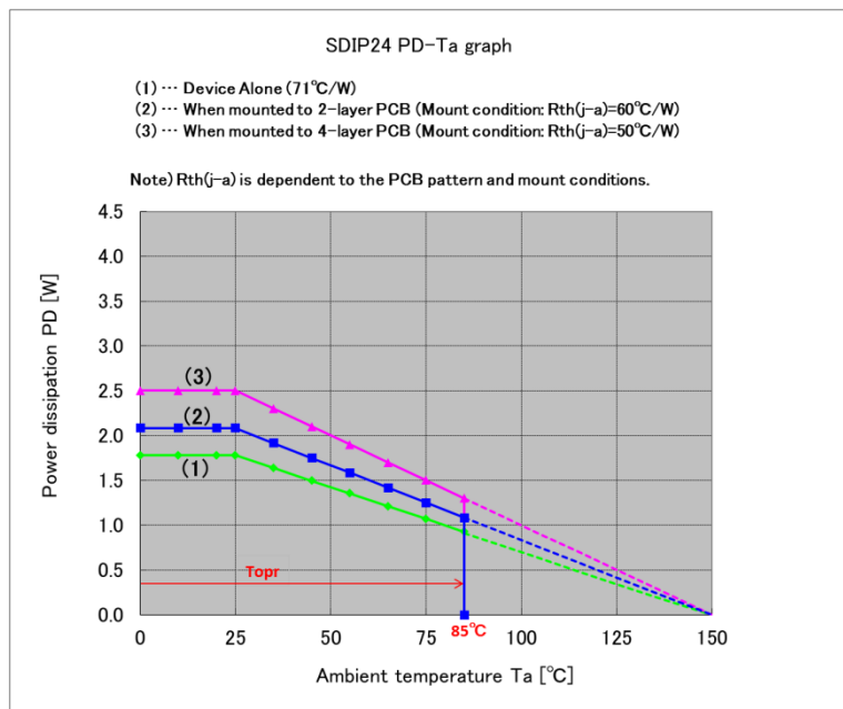
図 7 PD - Ta (パッケージの許容損失)
