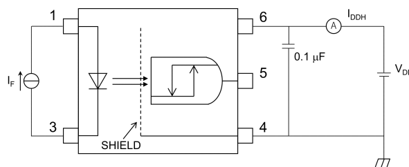
Fig. 12.1.4 I_{DDH} Test Circuit
