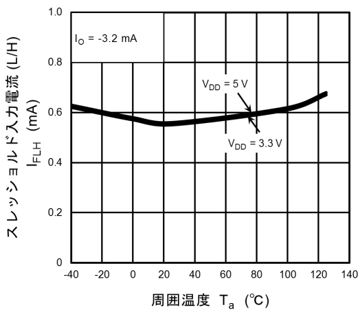
図 12.2.9 I_{FLH} - T_a
