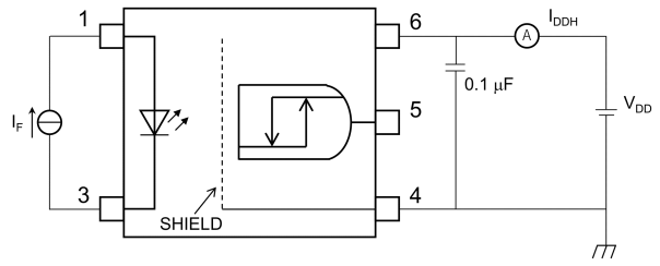
図 12.1.4 I_{DDH} 測定回路
