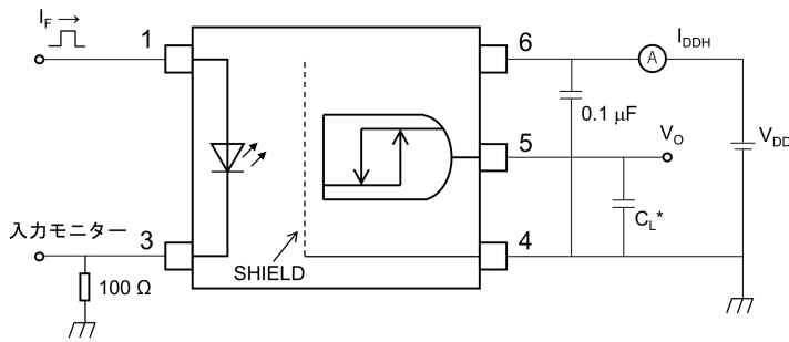
図 12.1.6 伝搬遅延時間測定回路, 波形
