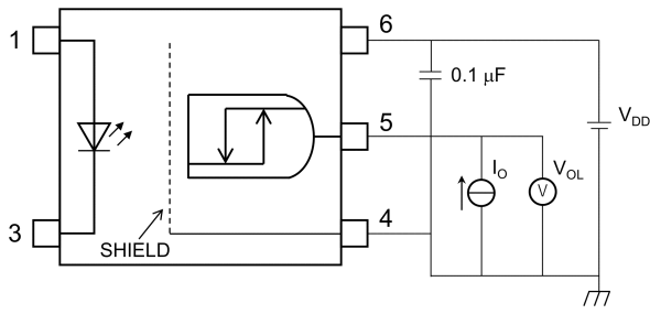
図 12.1.1 V_{OL} 測定回路
