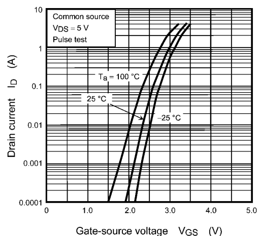
Fig. 8.2 I_D - V_{GS}
