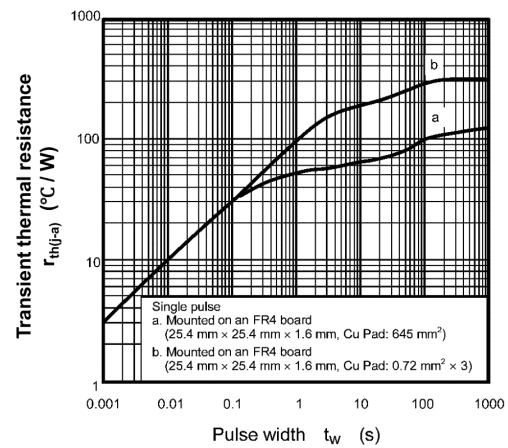
Fig. 8.12 r_{th(j-a)} - t_w
