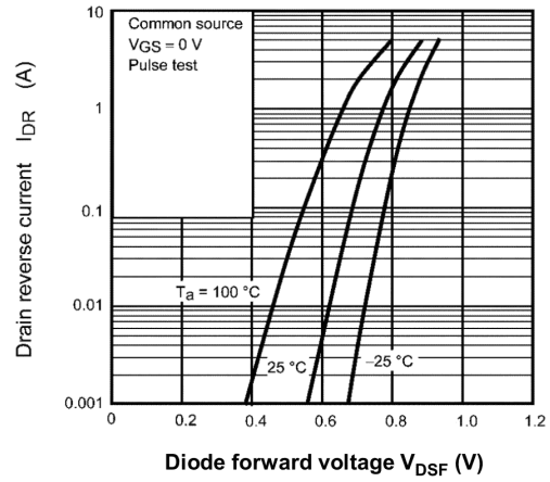
Fig. 8.8 I_{DR} - V_{DSF}
