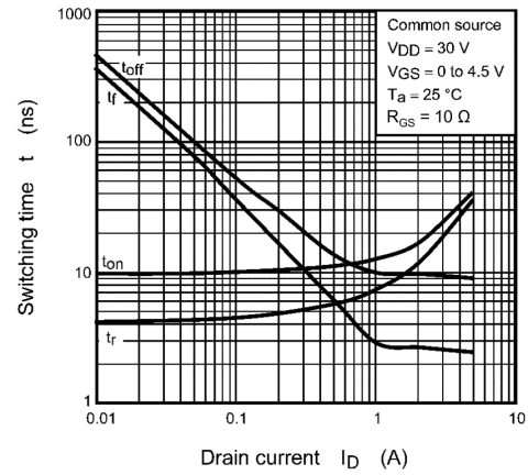
Fig. 8.10 t - I_D
