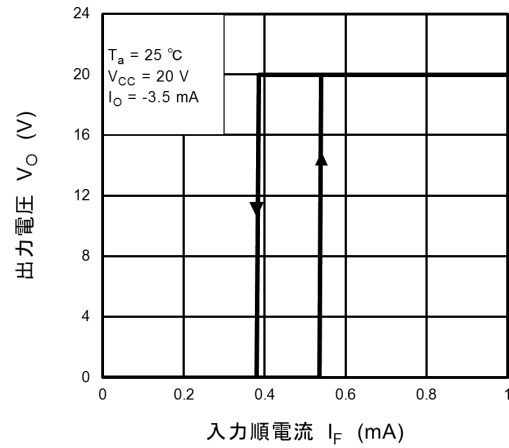
図 13.2.4 V_O - I_F(I_{HYS})
