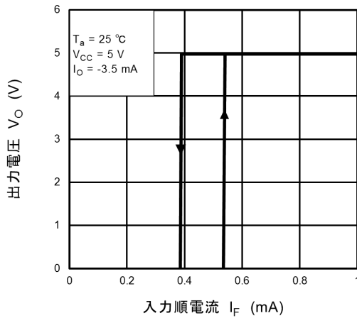
図 13.2.3 V_O - I_F(I_{HYS})
