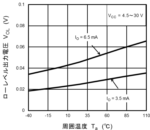
図 13.2.5 V_{OL} - T_a
