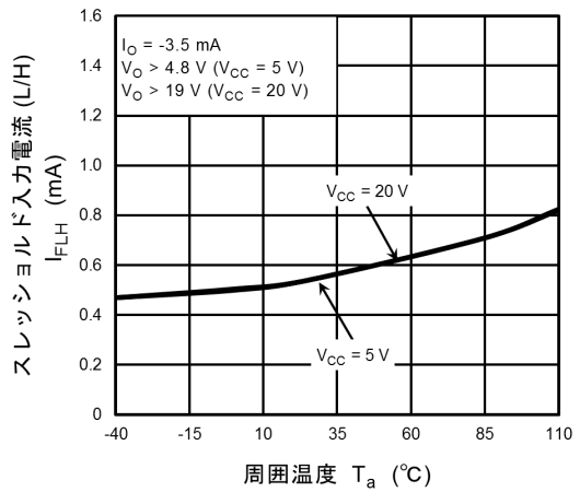
図 13.2.2 I_{FLH} - T_a
