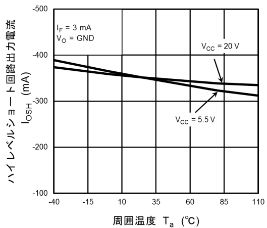
図 13.2.10 I_{osH} - T_a
