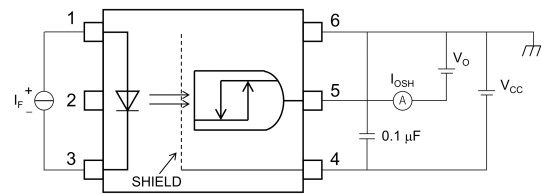
Fig. 13.1.6 I_{OH} Test Circuit
