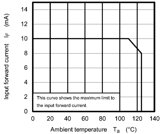
Fig. 13.2.2 I_F - T_a
