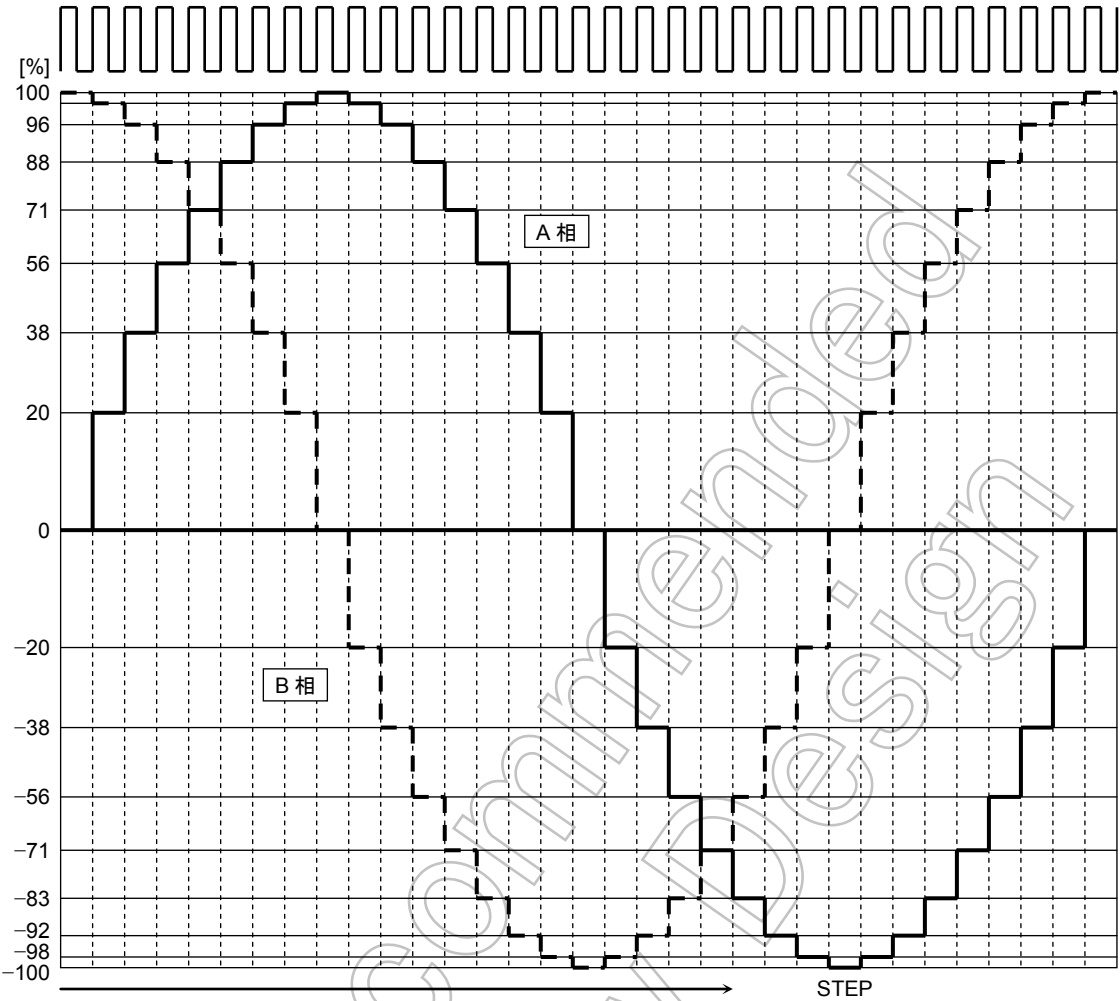
(7) 2W1-2 相励磁
