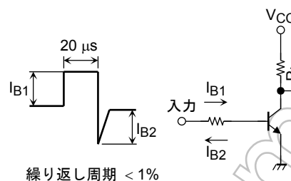
図 1 スイッチング時間測定回路
