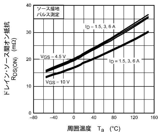
図 8.7 R_{DS(ON)} - T_a
