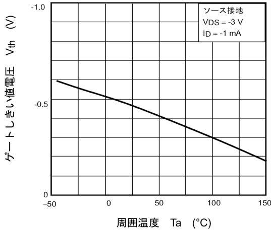
図 7.7 V_{th} - T_a
