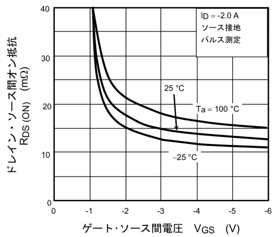
図 7.4 R_{DS(ON)} - V_{GS}
