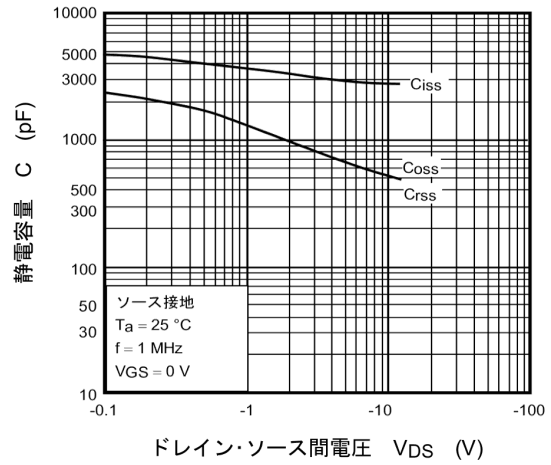
図 7.10 C - V_{DS}
