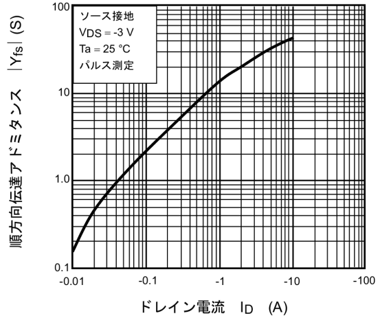
図 7.8 |Y_{fs}| - I_D
