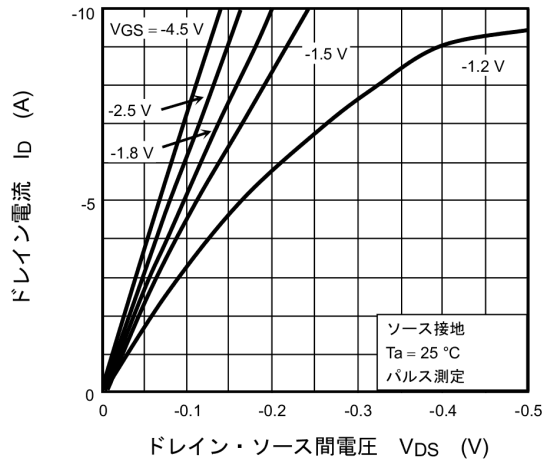
図 7.1 I_D - V_{DS}
