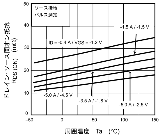
図 7.6 R_{DS(ON)} - T_a
