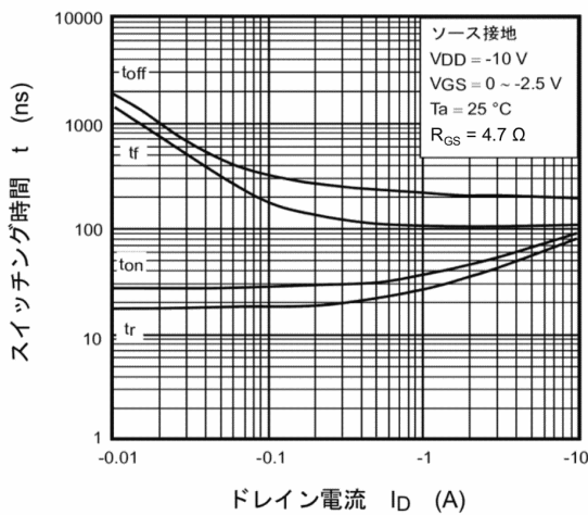
図 7.11 t - I_D
