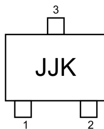
図 6.1 現品表示
