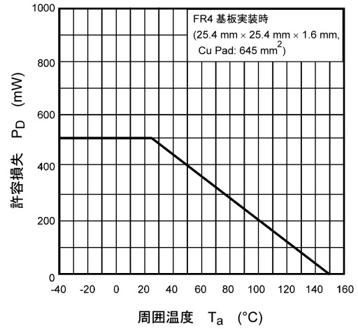
図 7.14 P_D - T_a
