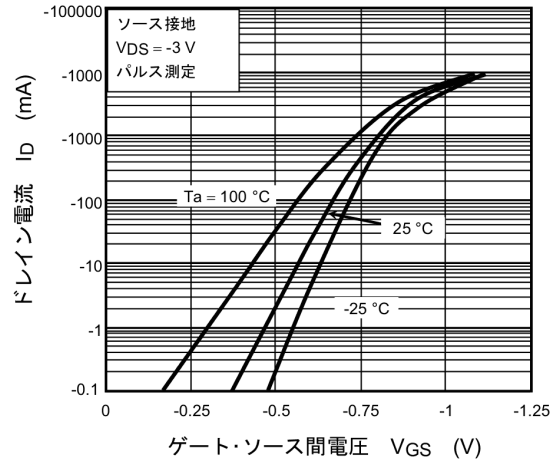
図 7.2 I_D - V_{GS}
