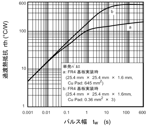
図 7.13 r_{th} - t_w
