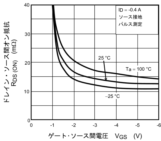
図 7.3 R_{DS(ON)} - V_{GS}
